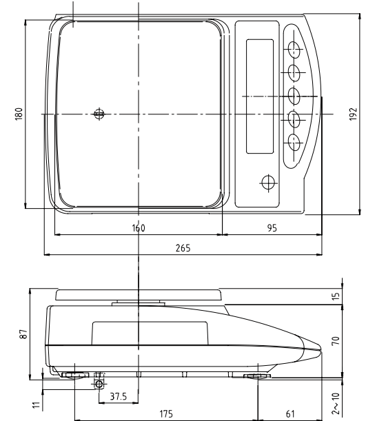
SJ-2200CE - SJ-12KCE
