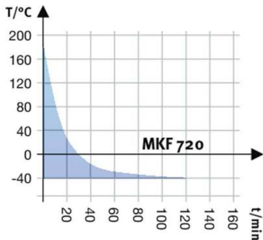
Кривая охлаждения
