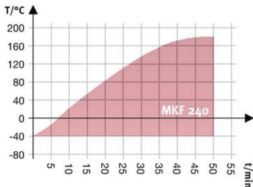
Кривая нагрева
